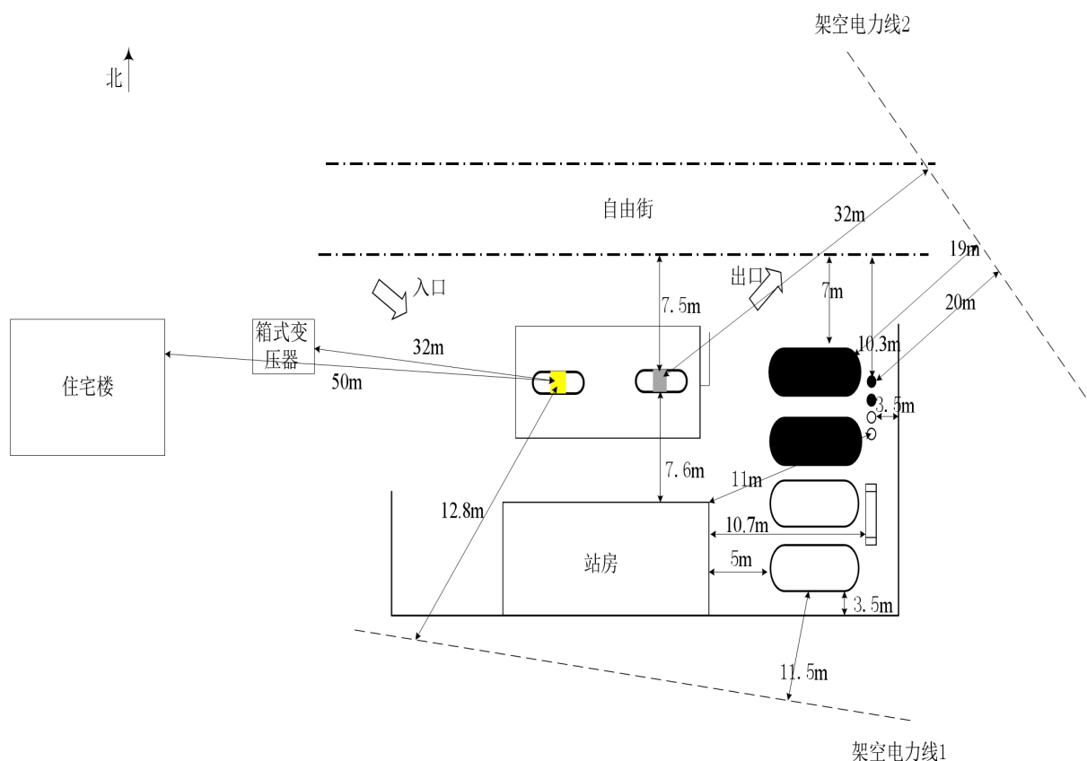
图2-1 周边环境及总平面布置情况示意图
