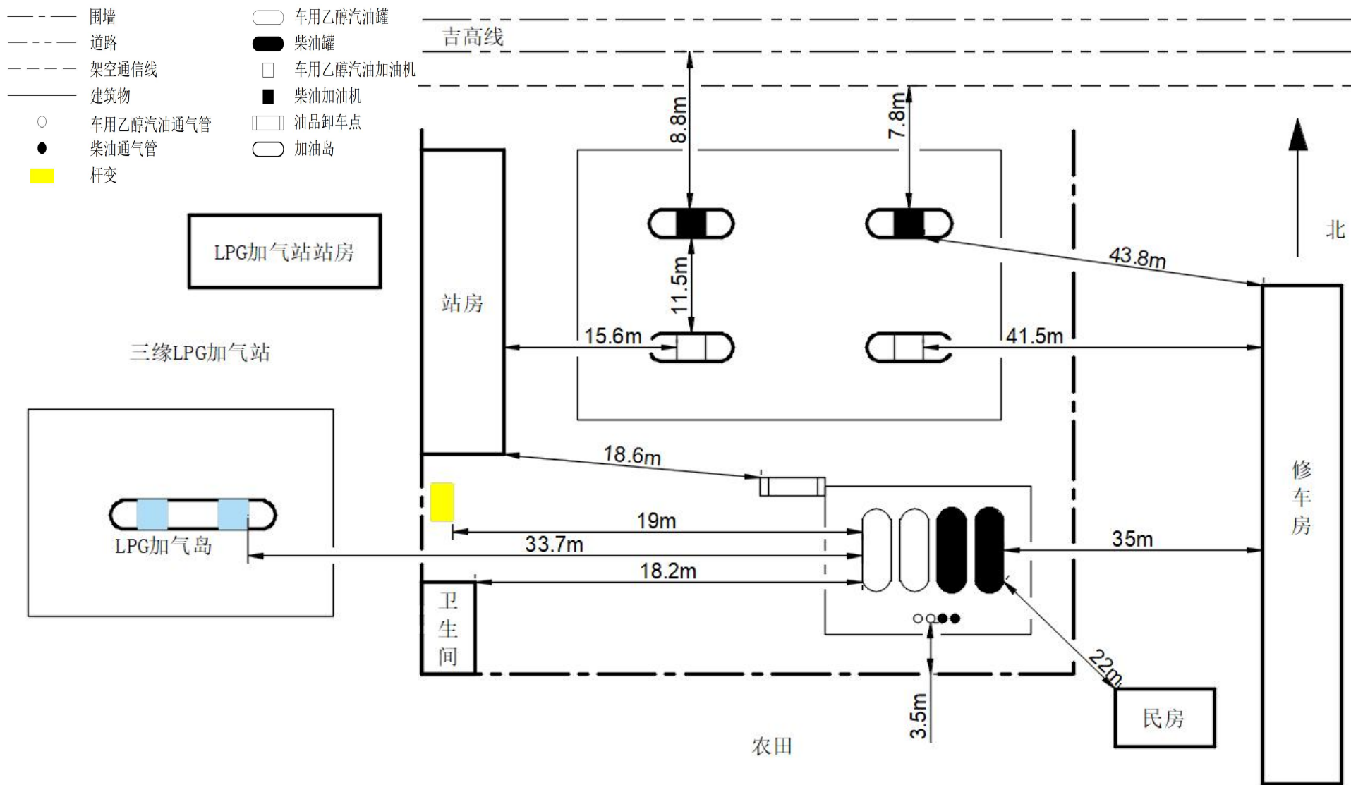
图 2-1 周边及总平面布置图
