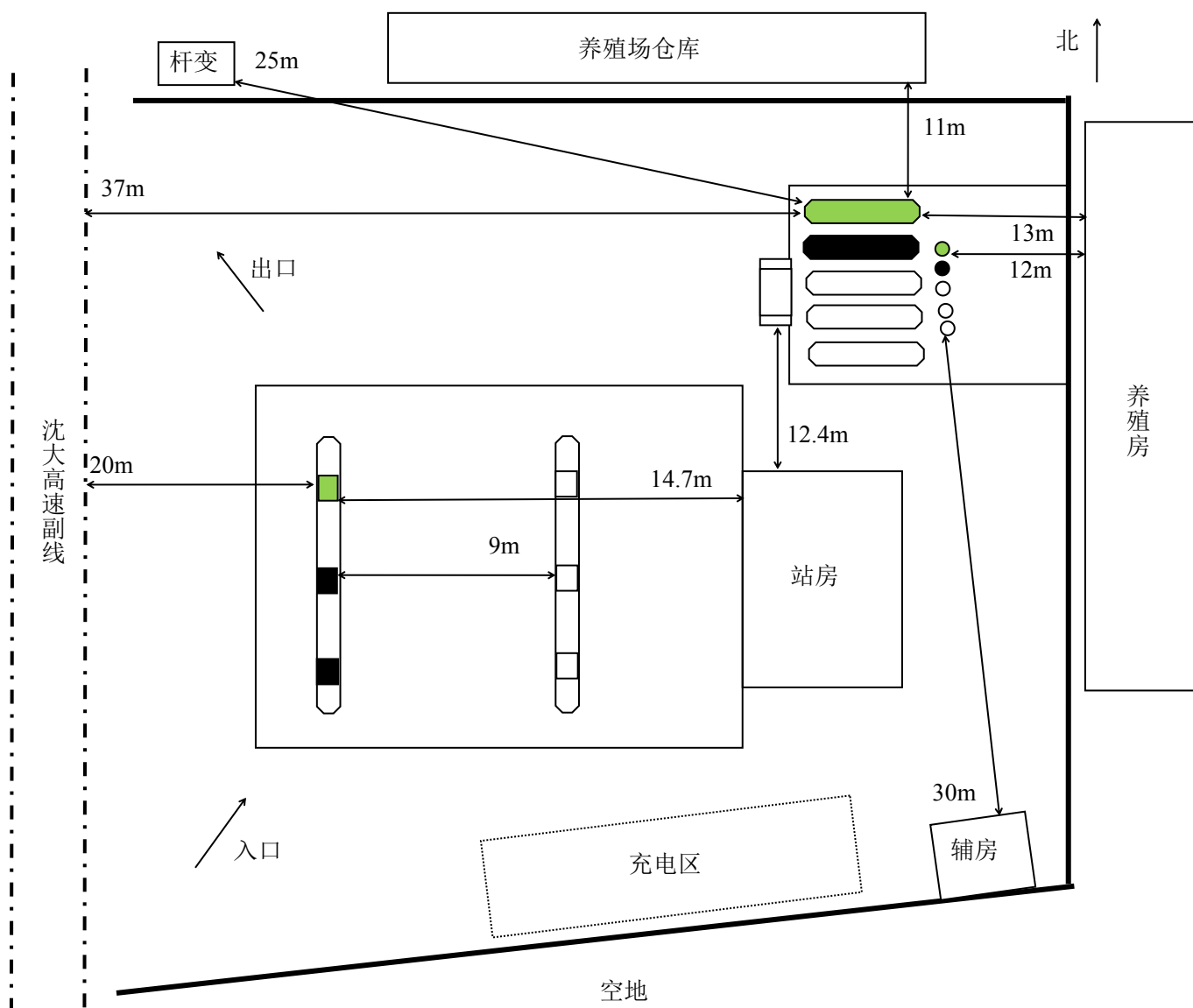
图 2-1 周边环境及总平面布置图
