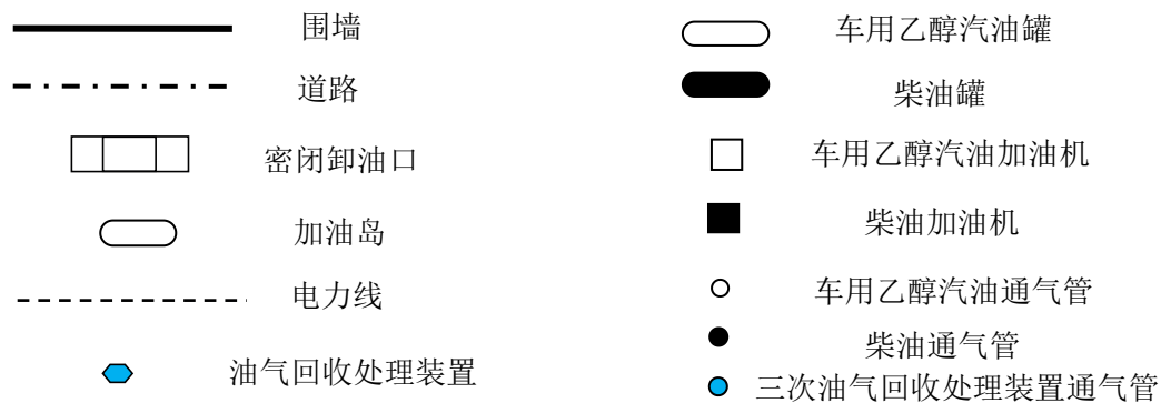
图 2.3-1 周边环境及总平面布置
