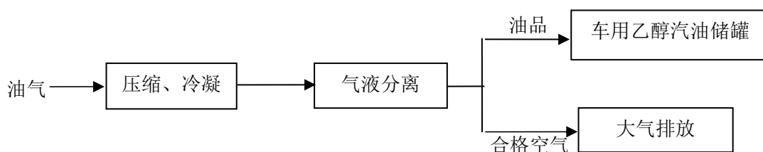
图 2.5-5 三次油气回收工艺流程框图
