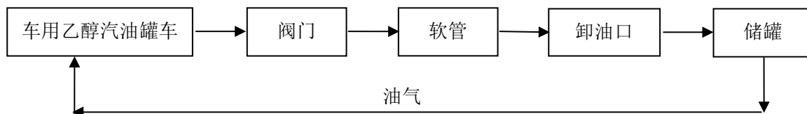
图 2.5-2 车用乙醇汽油卸油工艺流程框图
