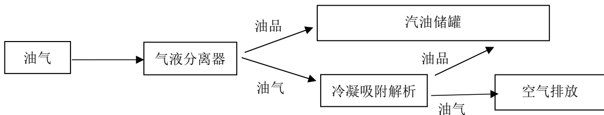
图 2.6-5 三次油气回收工艺流程框图
