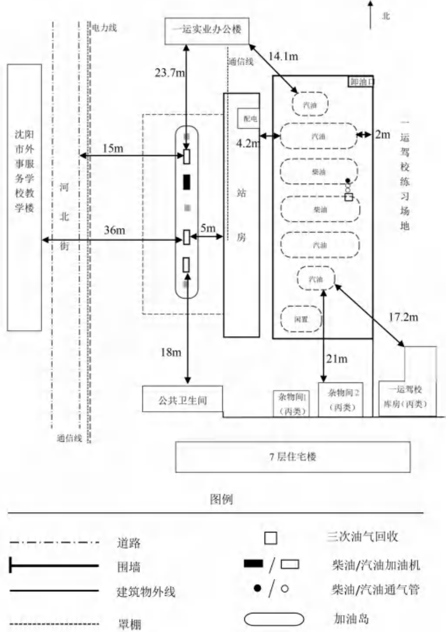
图 2.3-1 周边环境及总平面布置图
