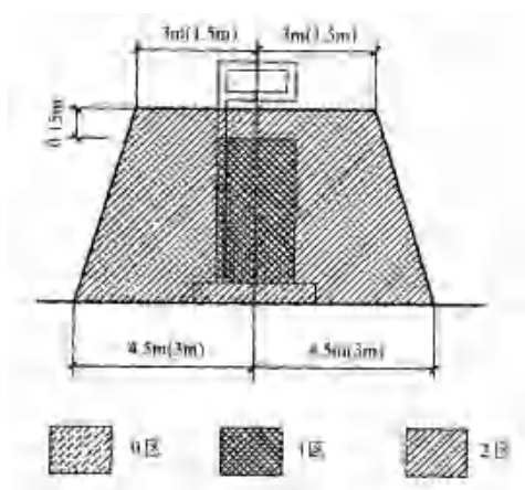
附图 1 汽油加油机爆炸危险区域划分
