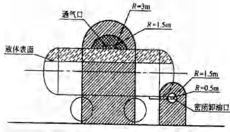
附图 2 油罐车卸汽油时爆炸危险区域划分
