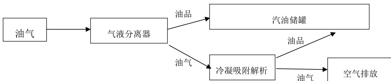
图 2-6 汽油三次油气回收工艺流程图
