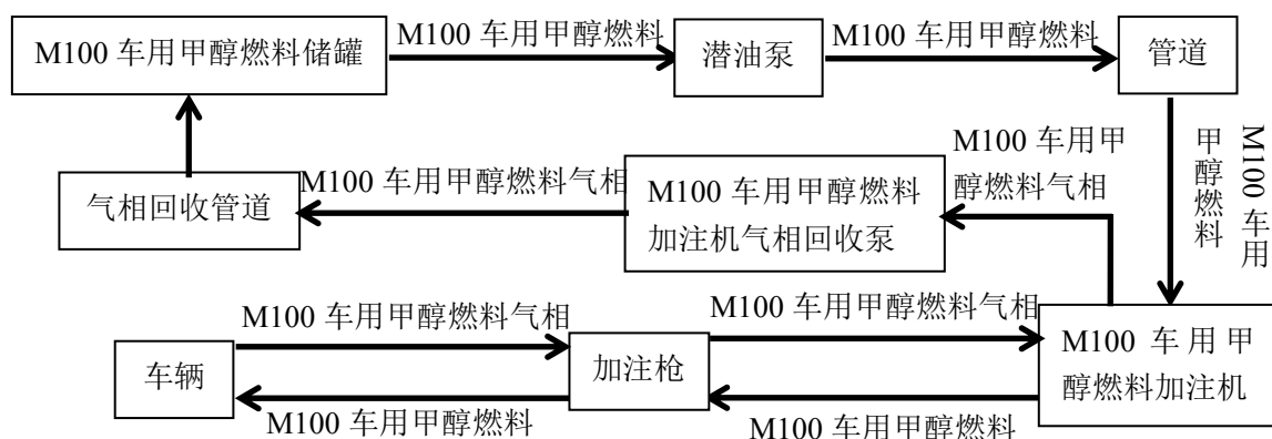
图 2.5-2 M100 车用甲醇燃料加液工艺流程图
