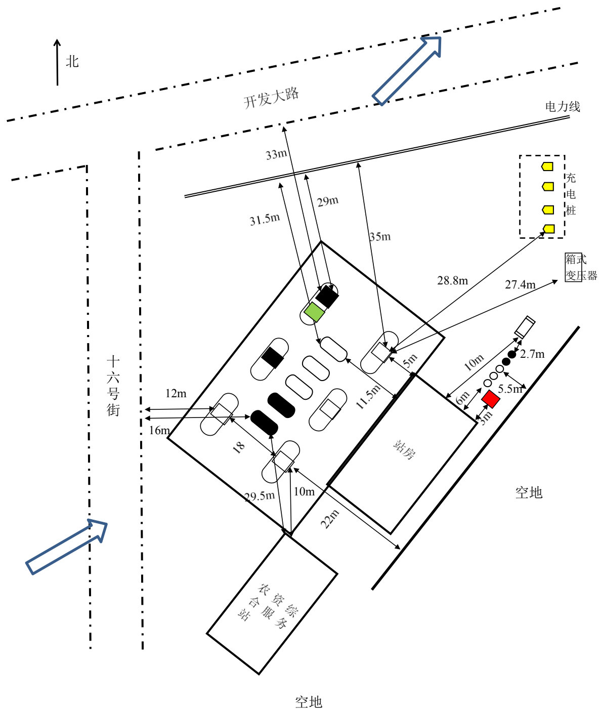
图 2.3-1 周边环境及总平面布置图
