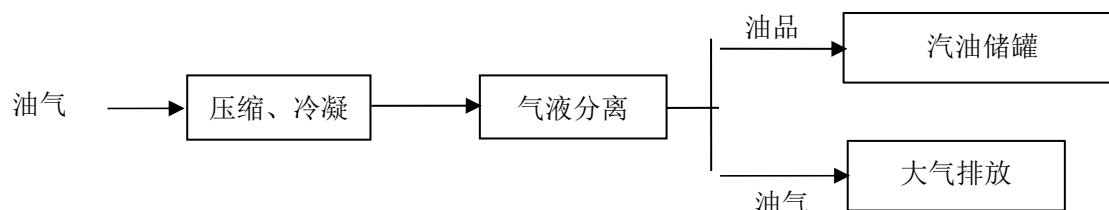
图 2-6 汽油三次油气回收工艺流程框图
