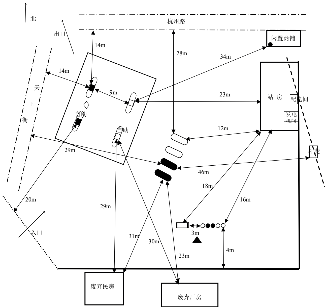
图 2-1 周边及总平面布置图
