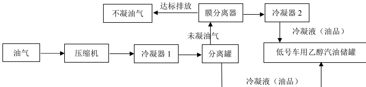
图 2-4 油气回收处理装置工艺流程框图（三次油气回收）
