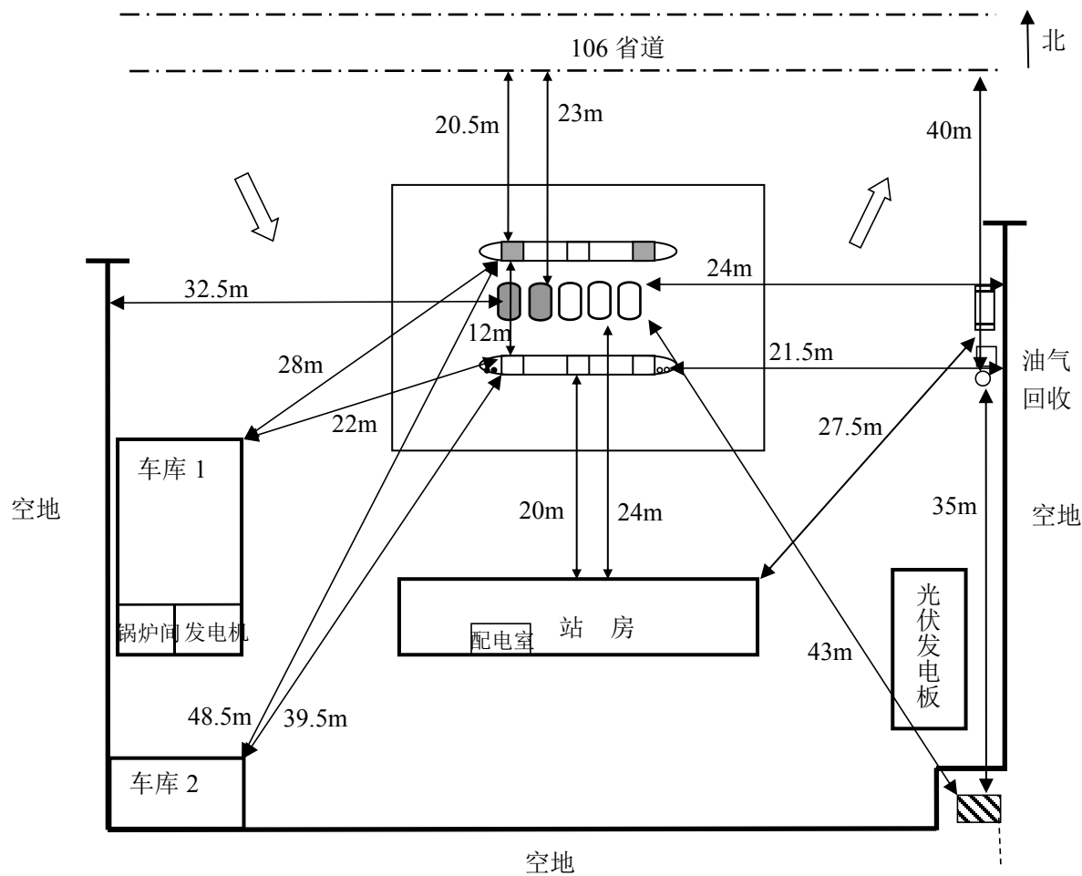
图 2-1 周边环境及总平面布置图
