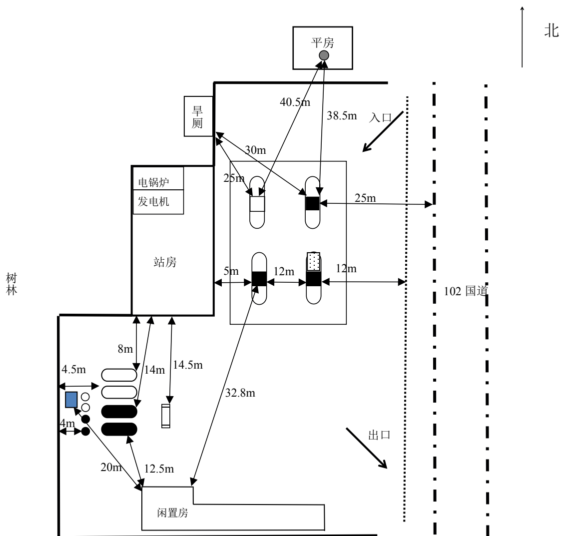
图 2-1 周边环境及总平面布置图
