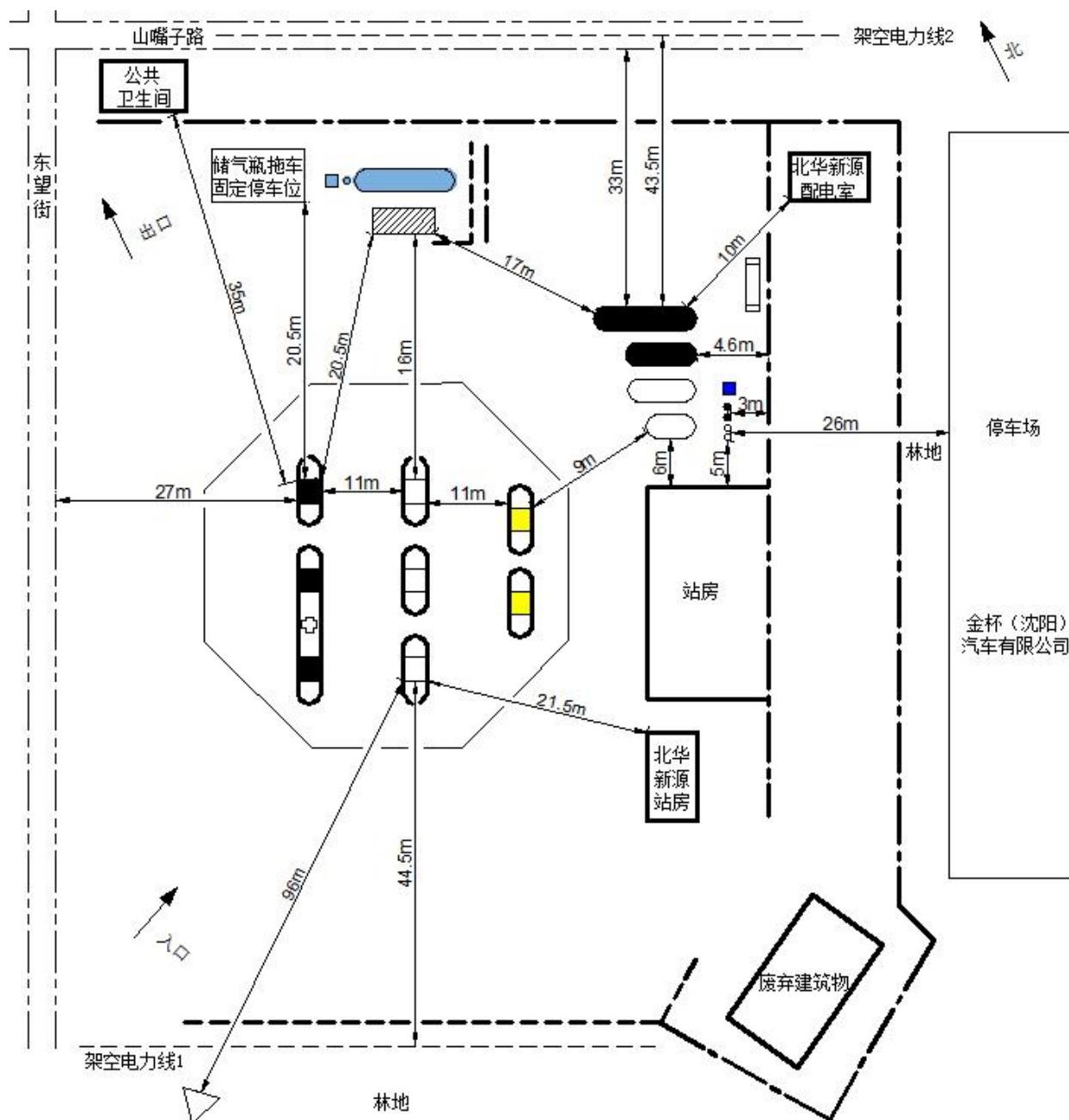
图 2-1 周边及总平面布置图
