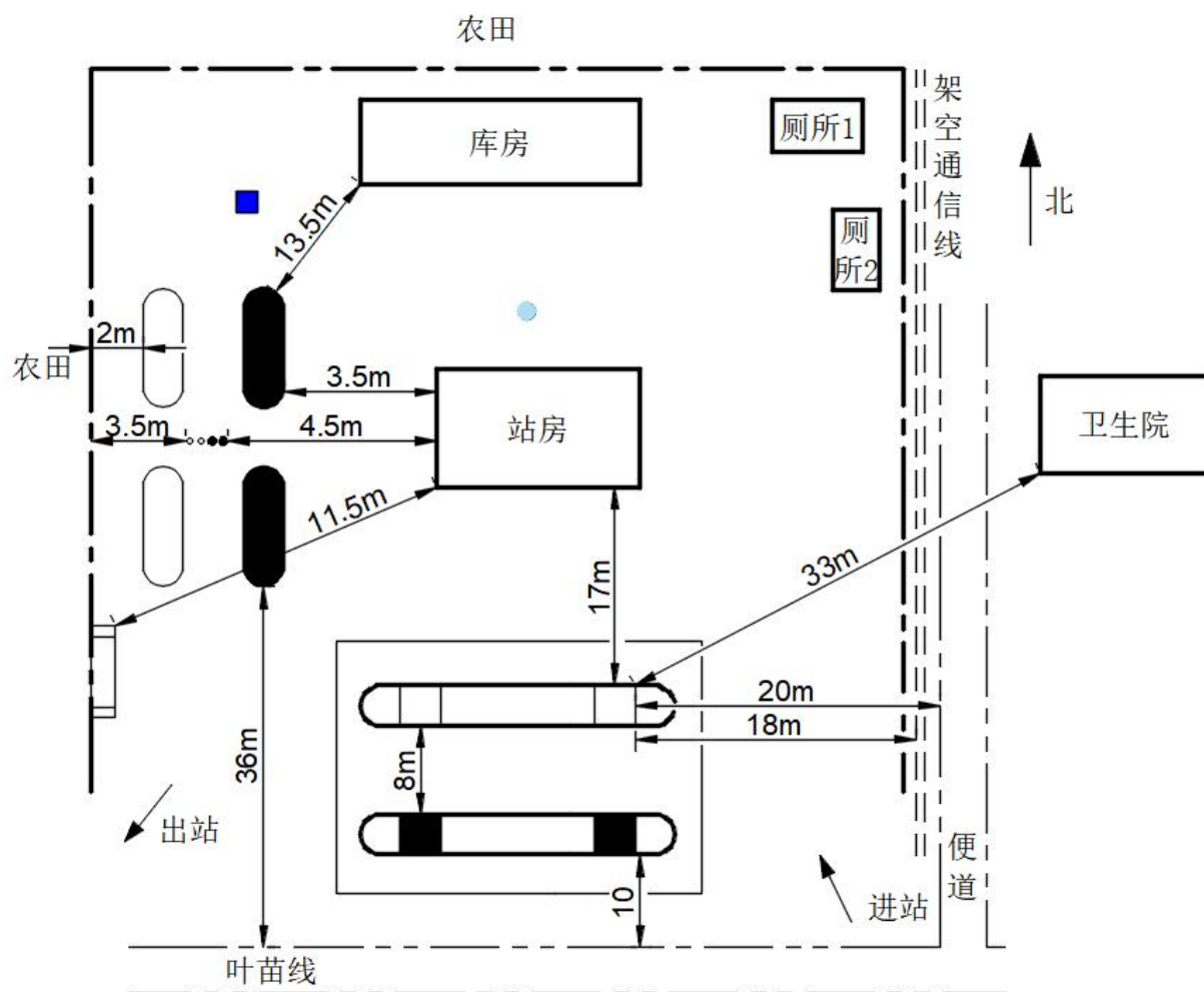
图 2-1 周边及总平面布置图
