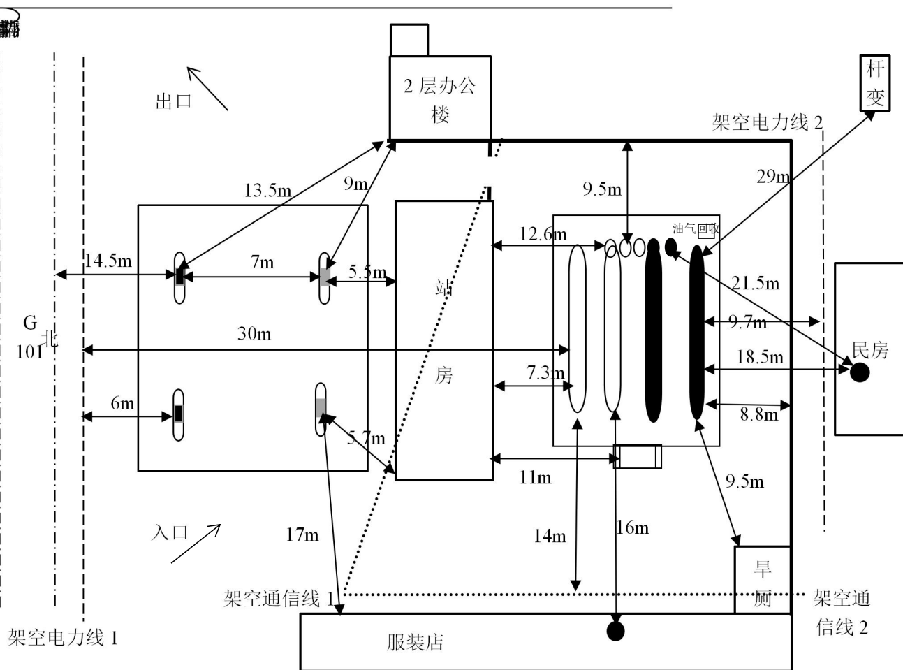
图 2.4-2 周边环境及总平面布置图
