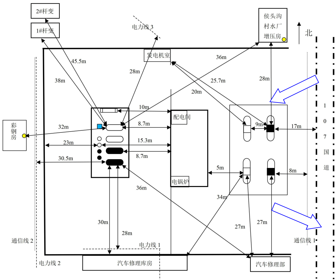
图 2.3-1 周边环境及总平面布置图
