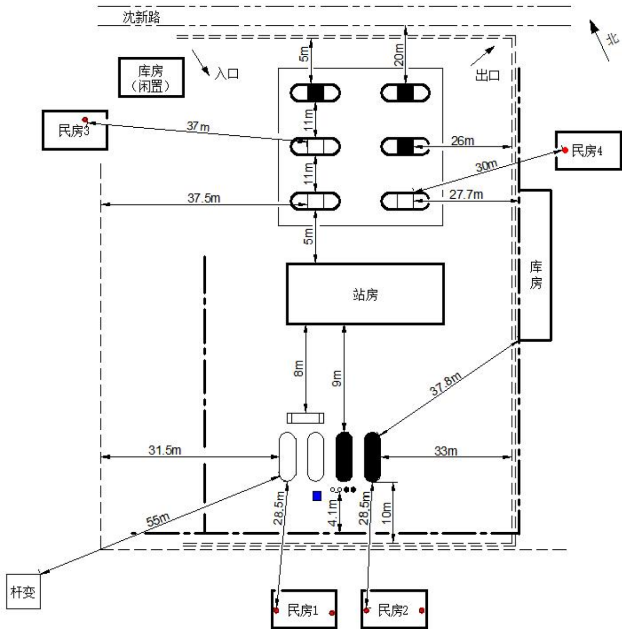
图 2-1 周边及总平面布置图
