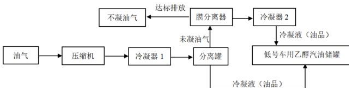
图 2-6 三次油气回收工艺流程图
