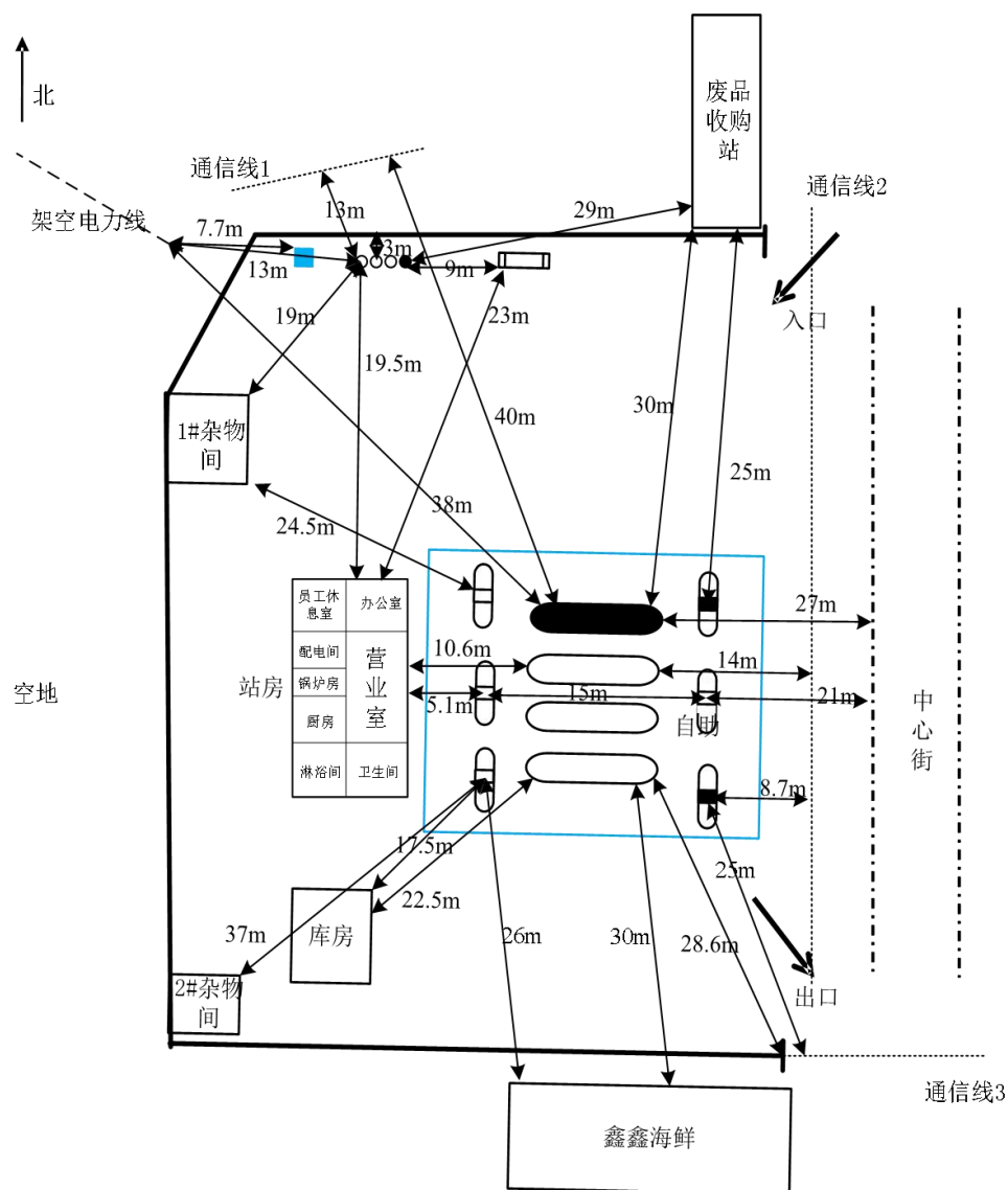
图2-1 周边及平面布置总图
