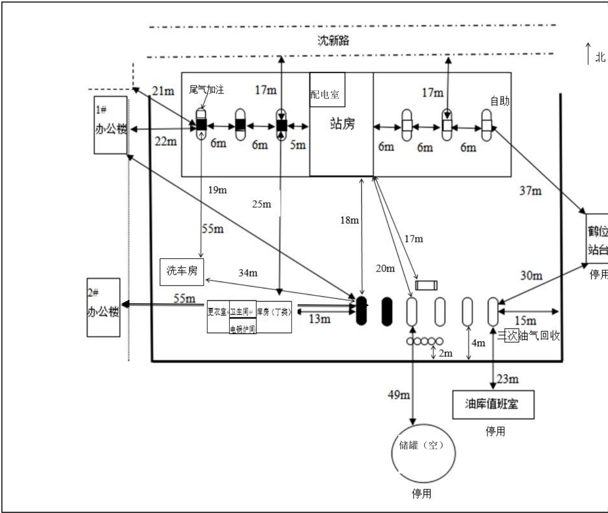
图 2.3-1 总平面布置图
