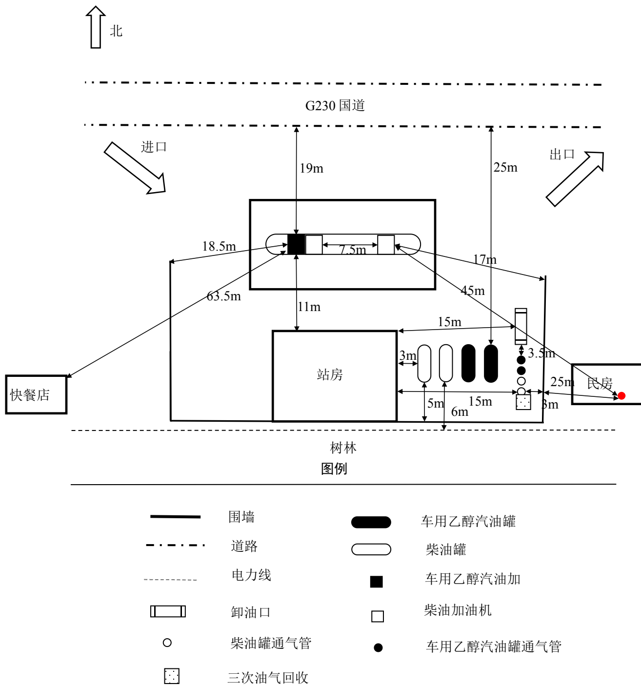
图 2.3-1 周边环境及总平面布置
