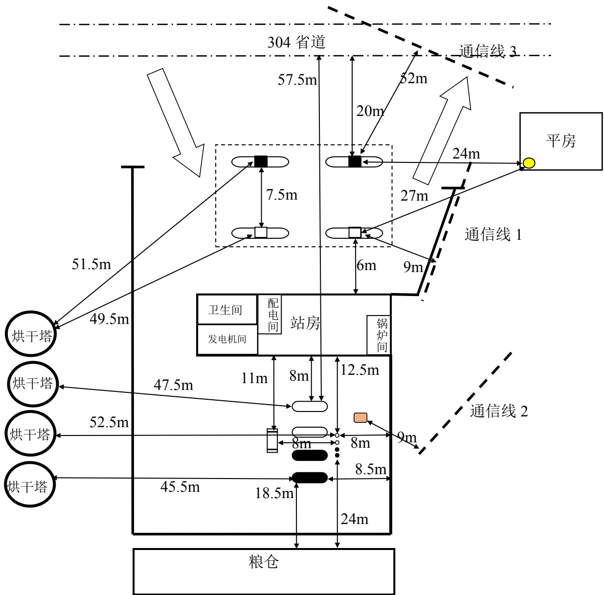
图 2.3-1 周边环境及总平面布置图 图例
