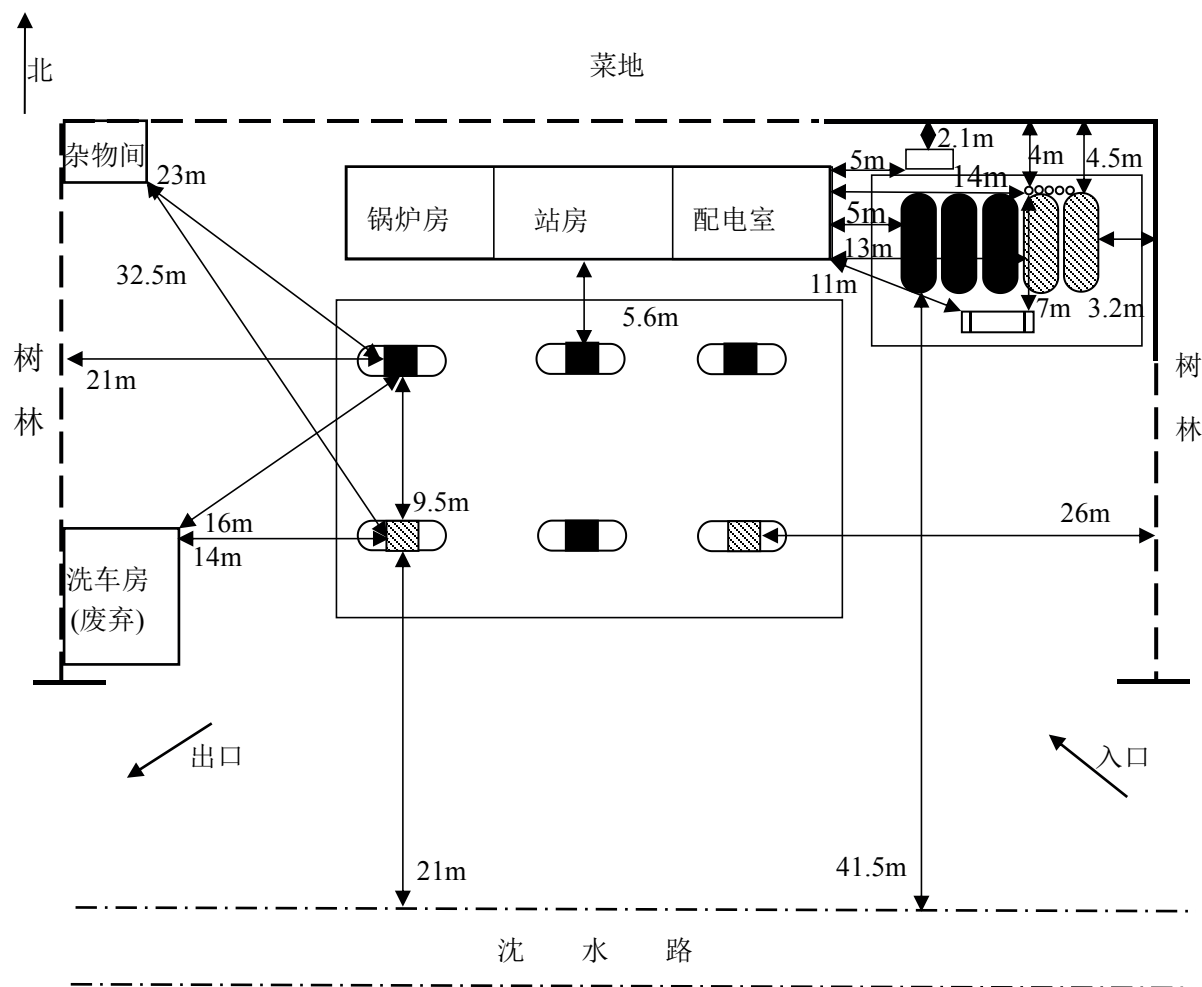
图 2-1 周边环境及总平面布置图
