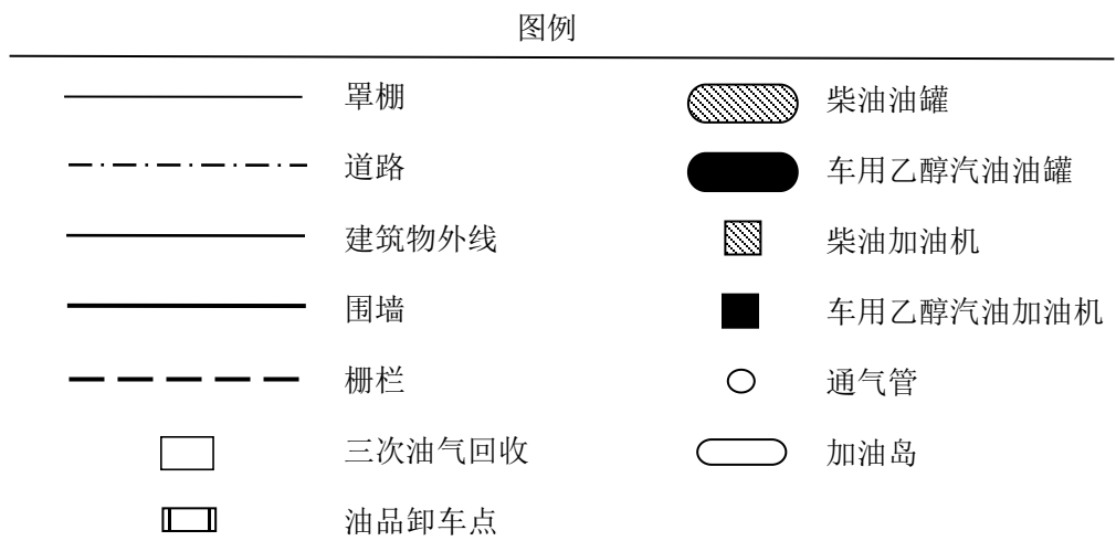
图 2.3-1 周边环境及总平面布置
