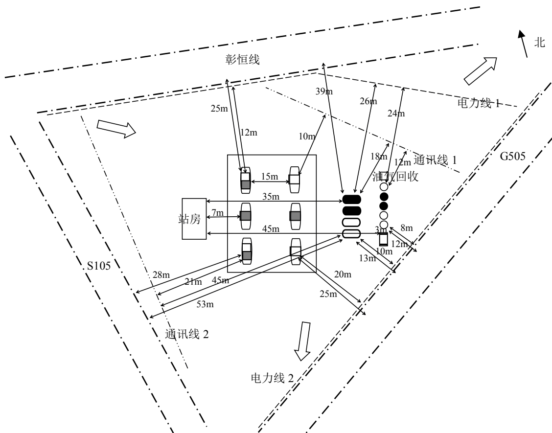
图 2-1 周边环境及总平面布置图
