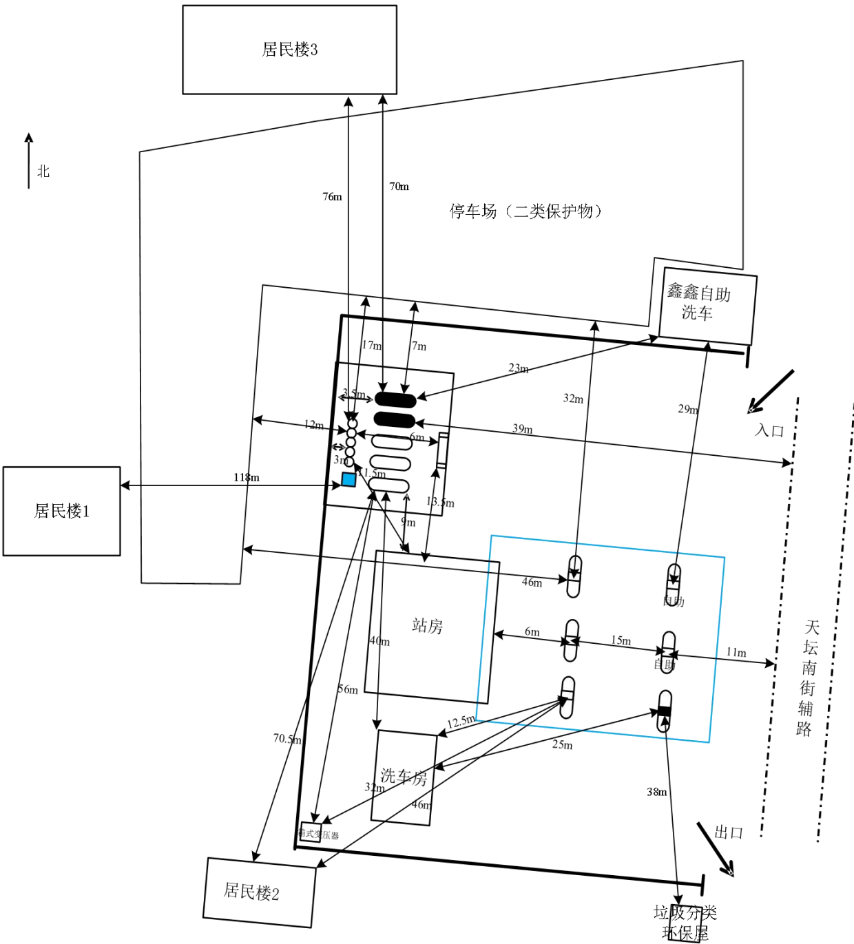
图2-1 周边及平面布置总图
