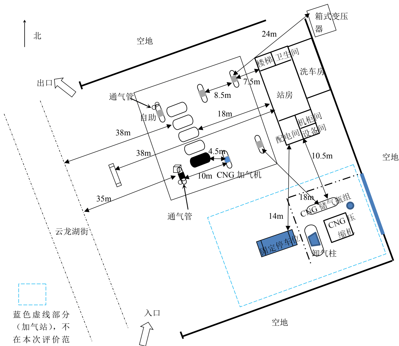
图 2-1 周边环境及总平面布置情况示意图
