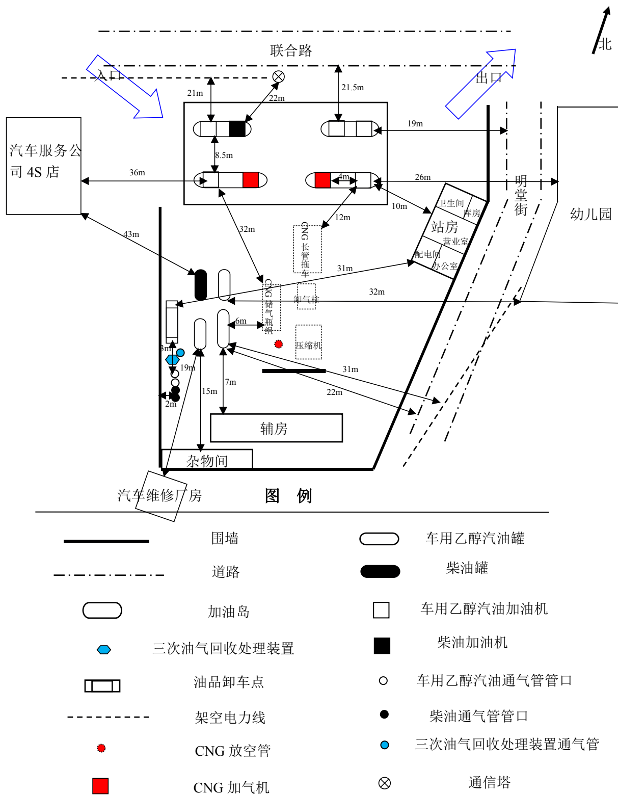
图 2.3-1 周边环境及总平面布置
