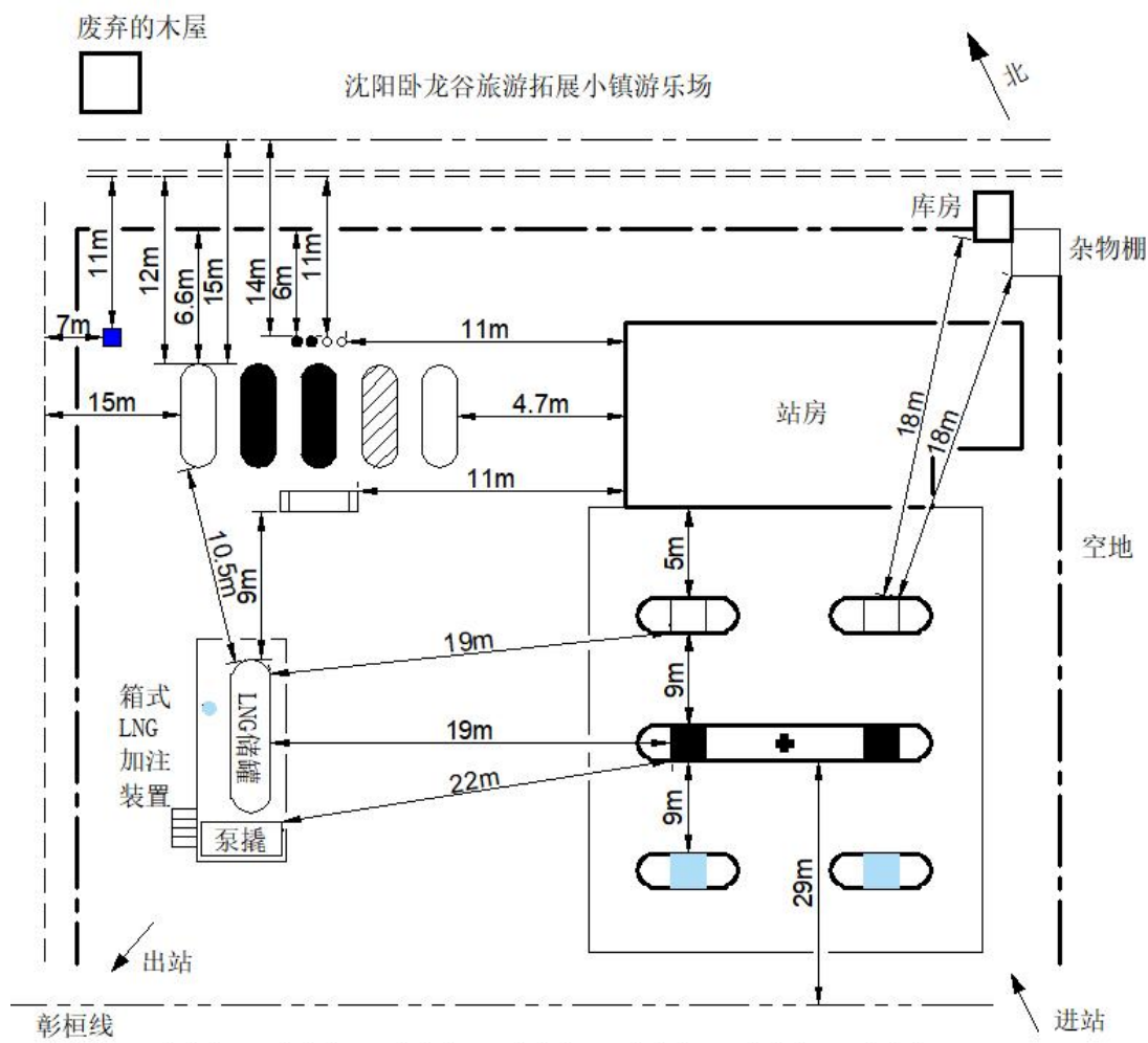
图 2-1 周边及总平面布置图
