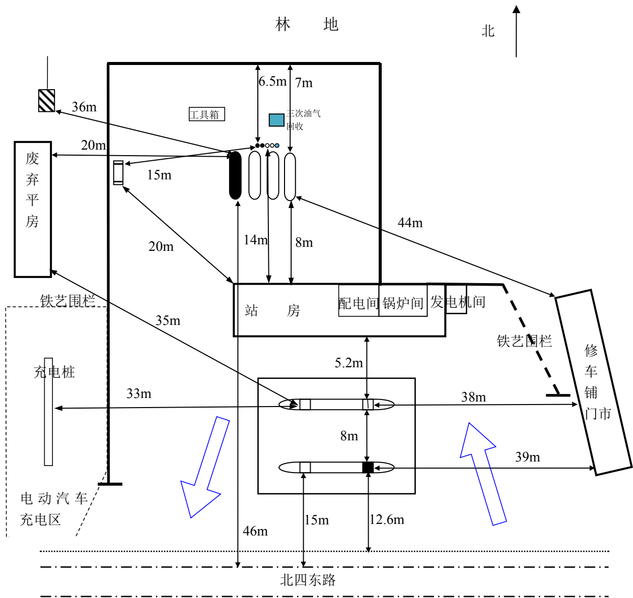
图 2.3-1 周边环境及总平面布置图
