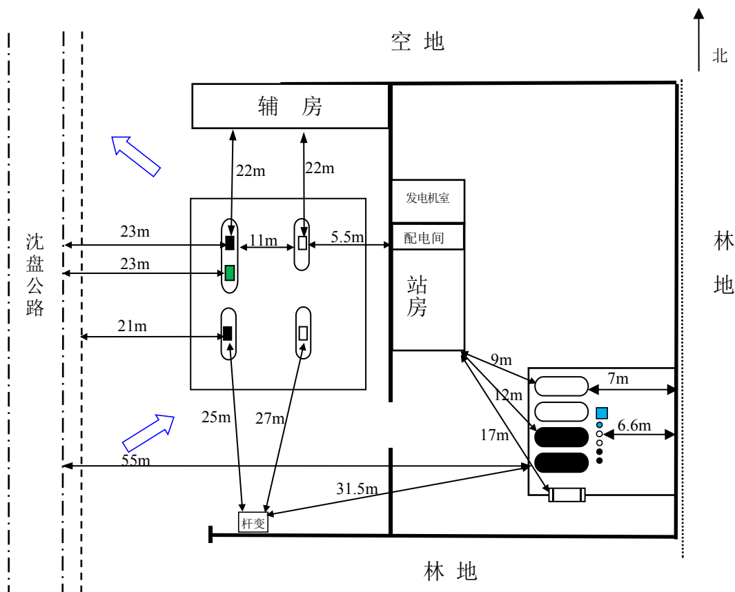
图 2.3-1 周边环境及总平面布置图
