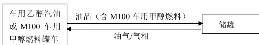
图 2-2 车用乙醇汽油或 M100 车用甲醇燃料卸油/液工艺流程框图（一次）
