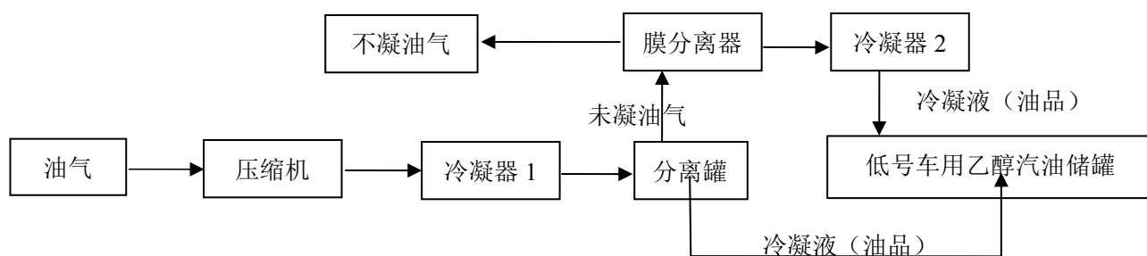
图 2-4 油气回收处理装置工艺流程框图（三次油气回收）
