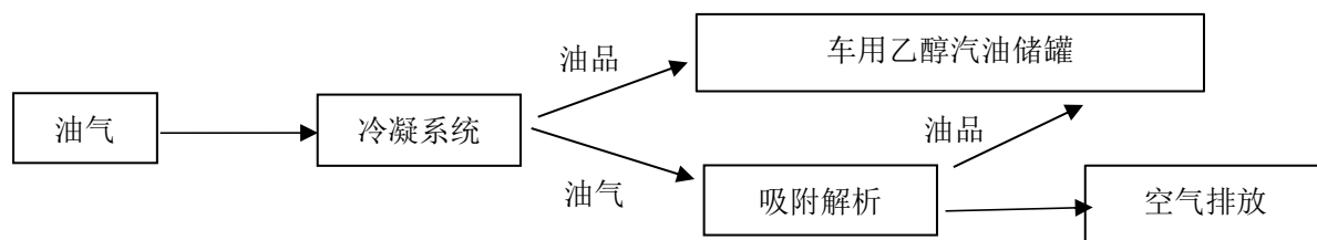
图 2-6 三次油气回收工艺流程框图
