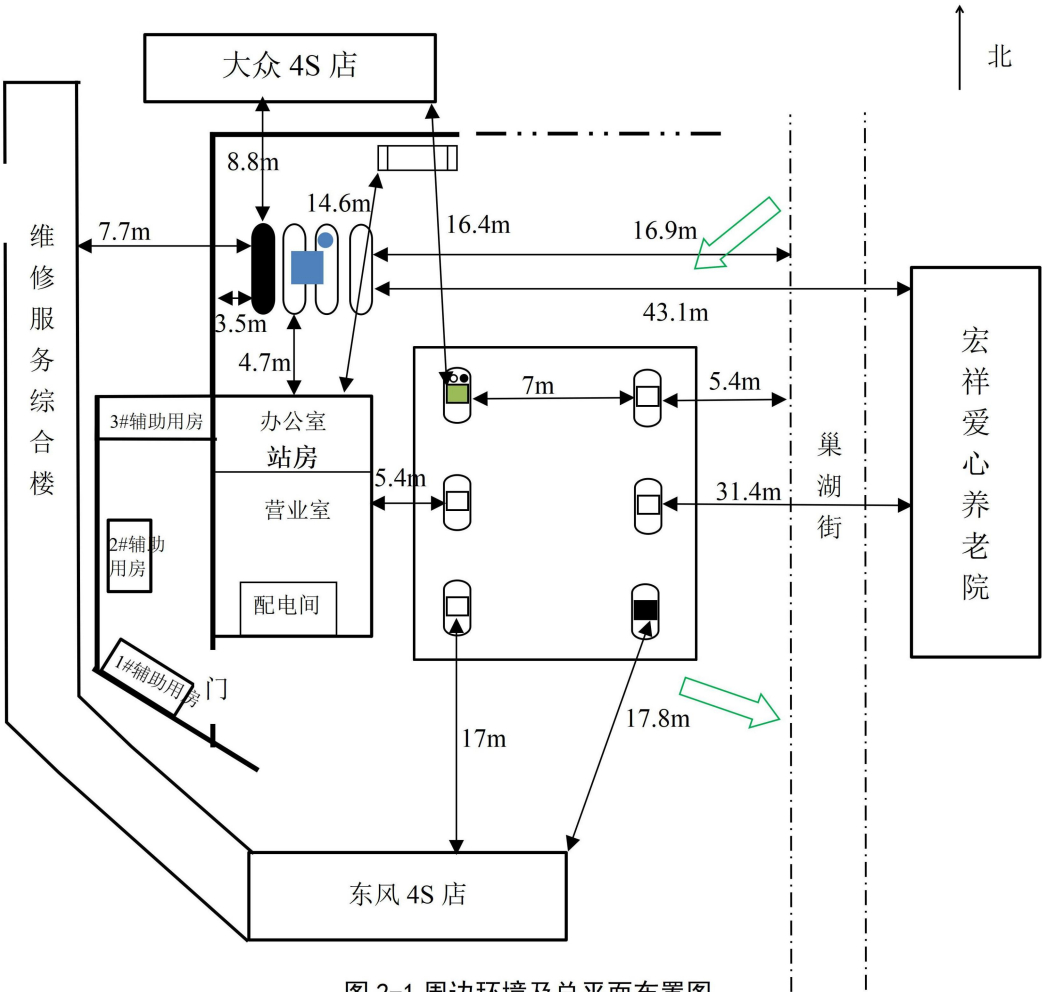
图 2-1 周边环境及总平面布置图
