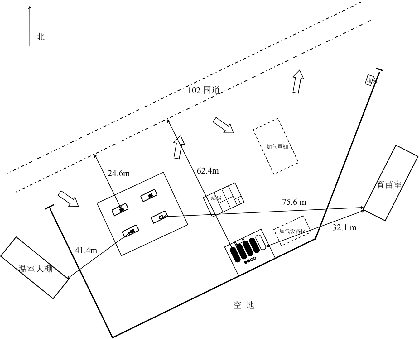
图 2.3-2 周边环境示意图
