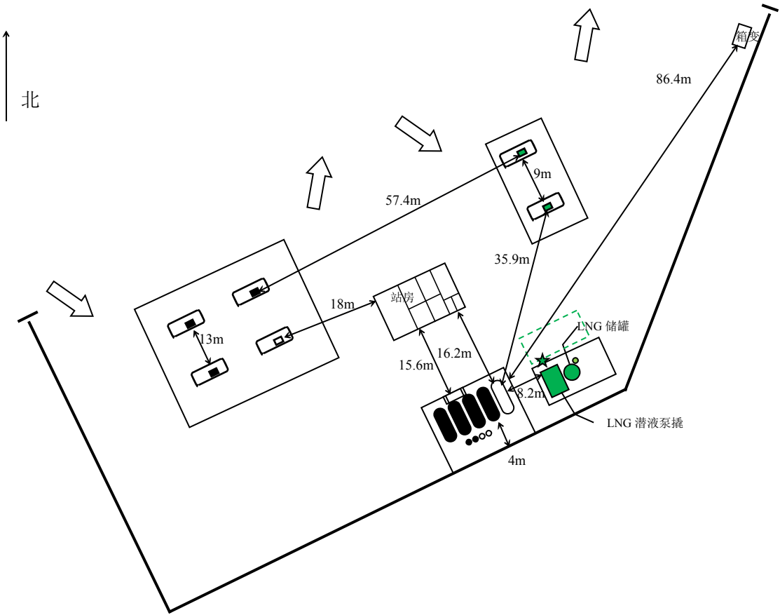
图 2.3-3 总平面布置图
