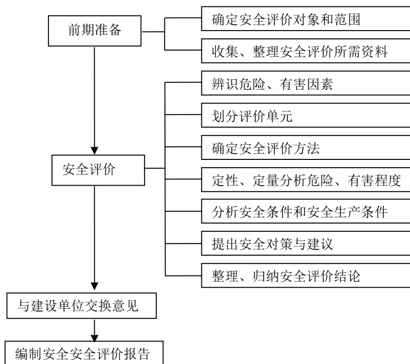
图 1.4-1 安全验收评价程序框图
