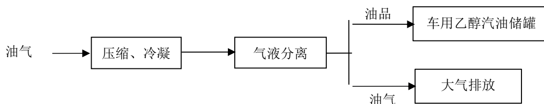
图 2-5 三次油气回收工艺流程框图
