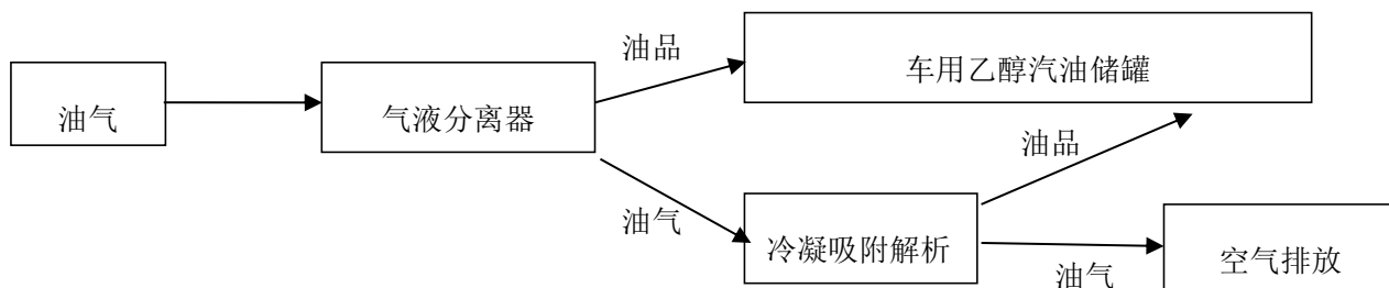
图 2-6 车用乙醇汽油三次油气回收工艺流程图
