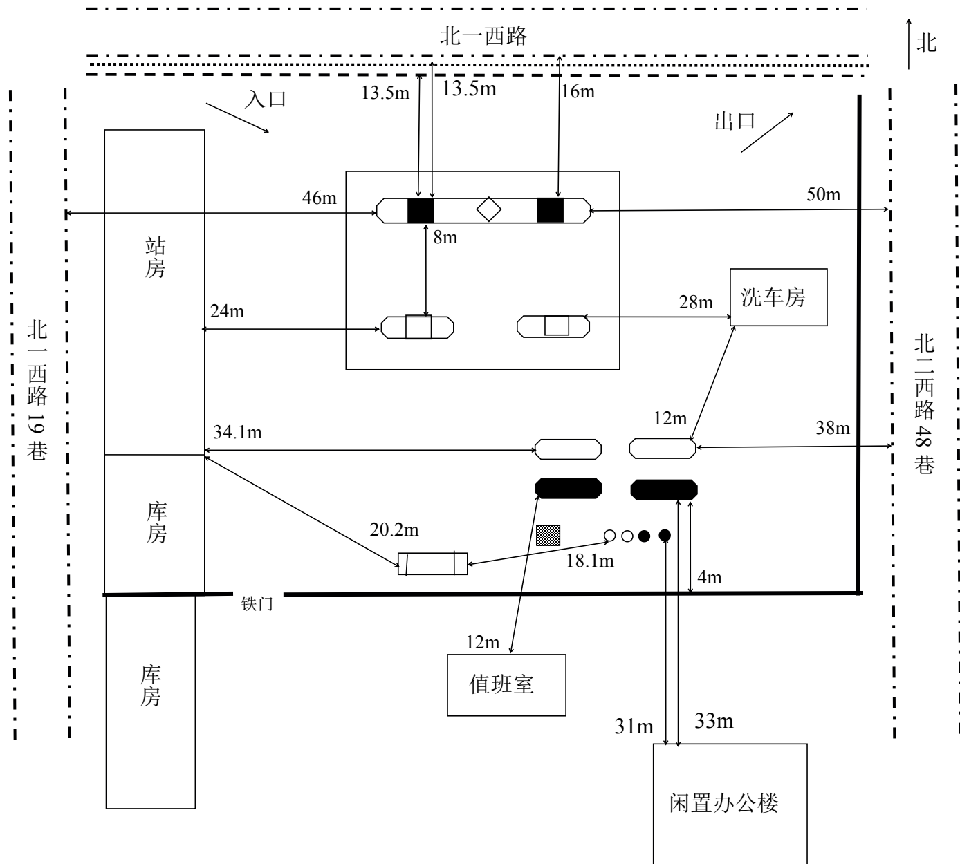
图 2-1 周边环境及总平面布置图
