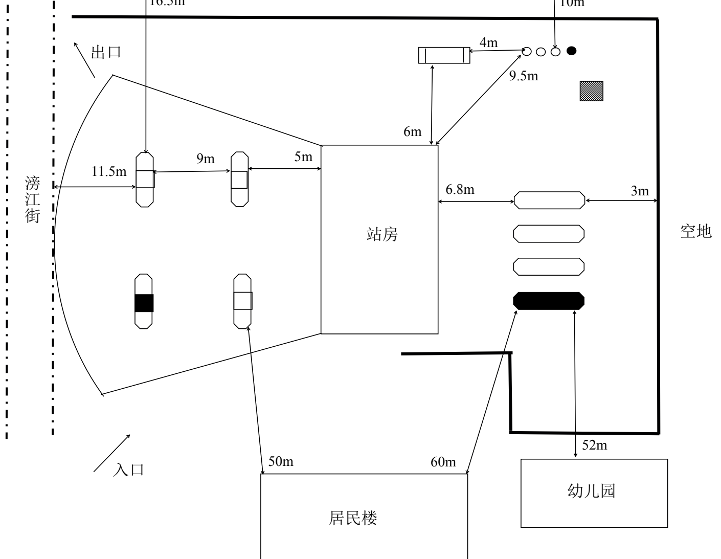
图 2-1 周边环境及总平面布置图
