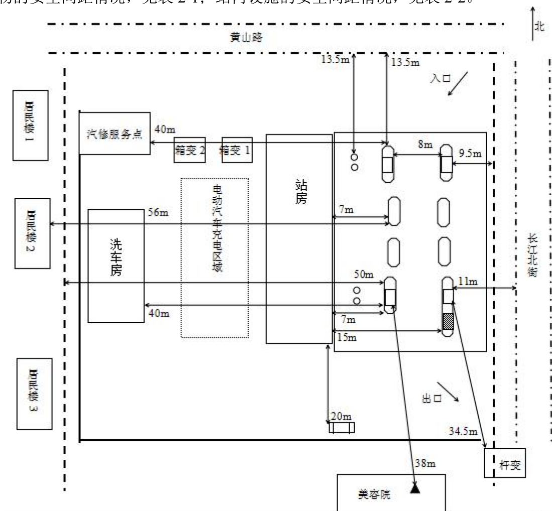
图 2-1 周边环境及总平面布置图
