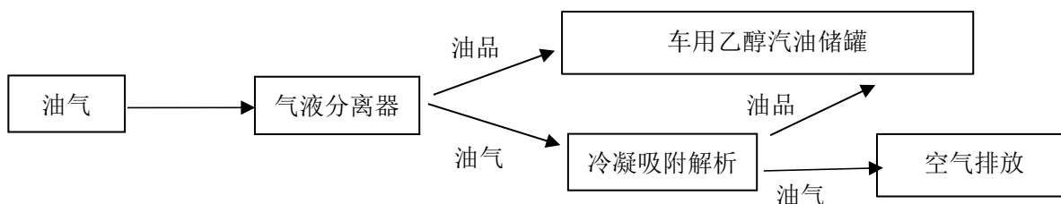
图 2-4 三次油气回收工艺流程框图
