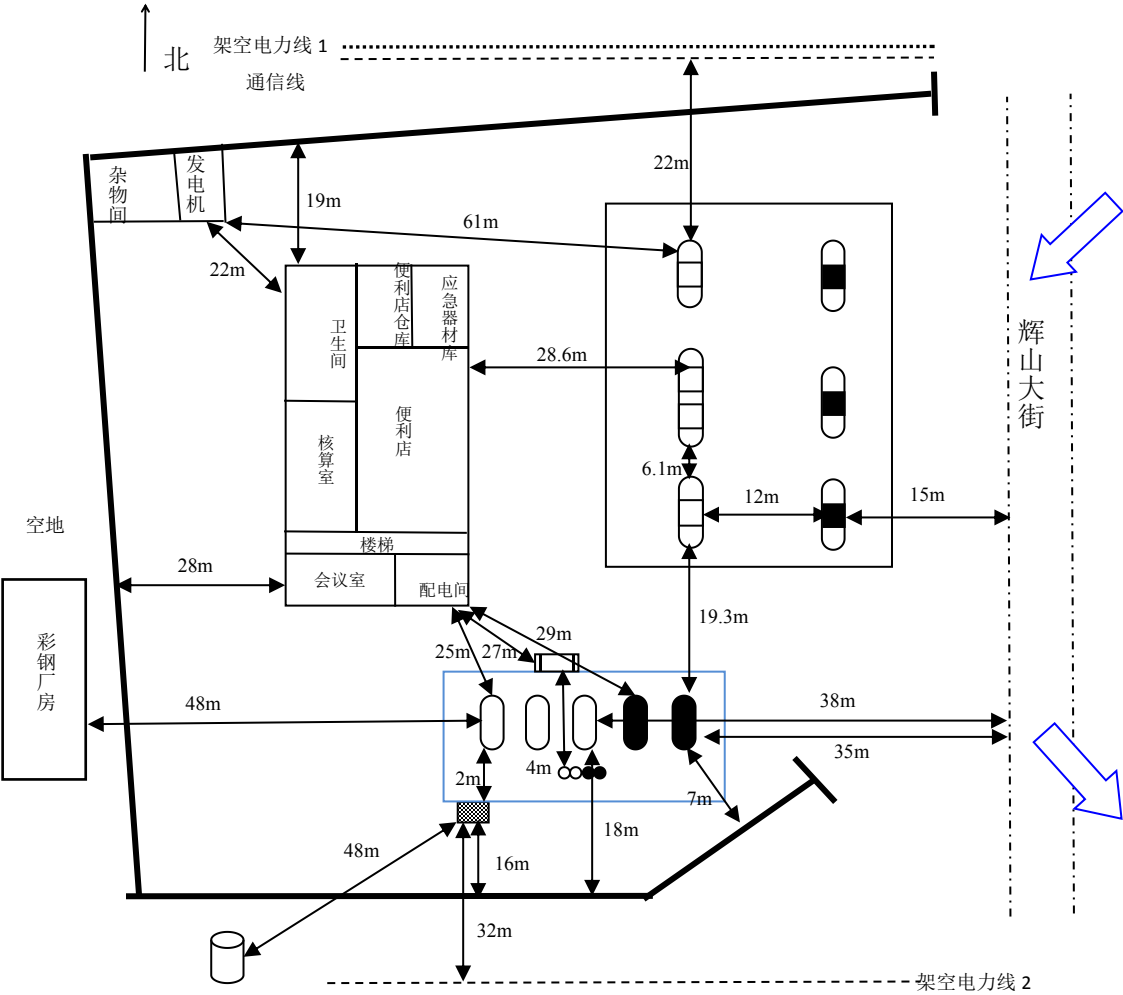
图 2-1 周边环境及总平面布置示意图
