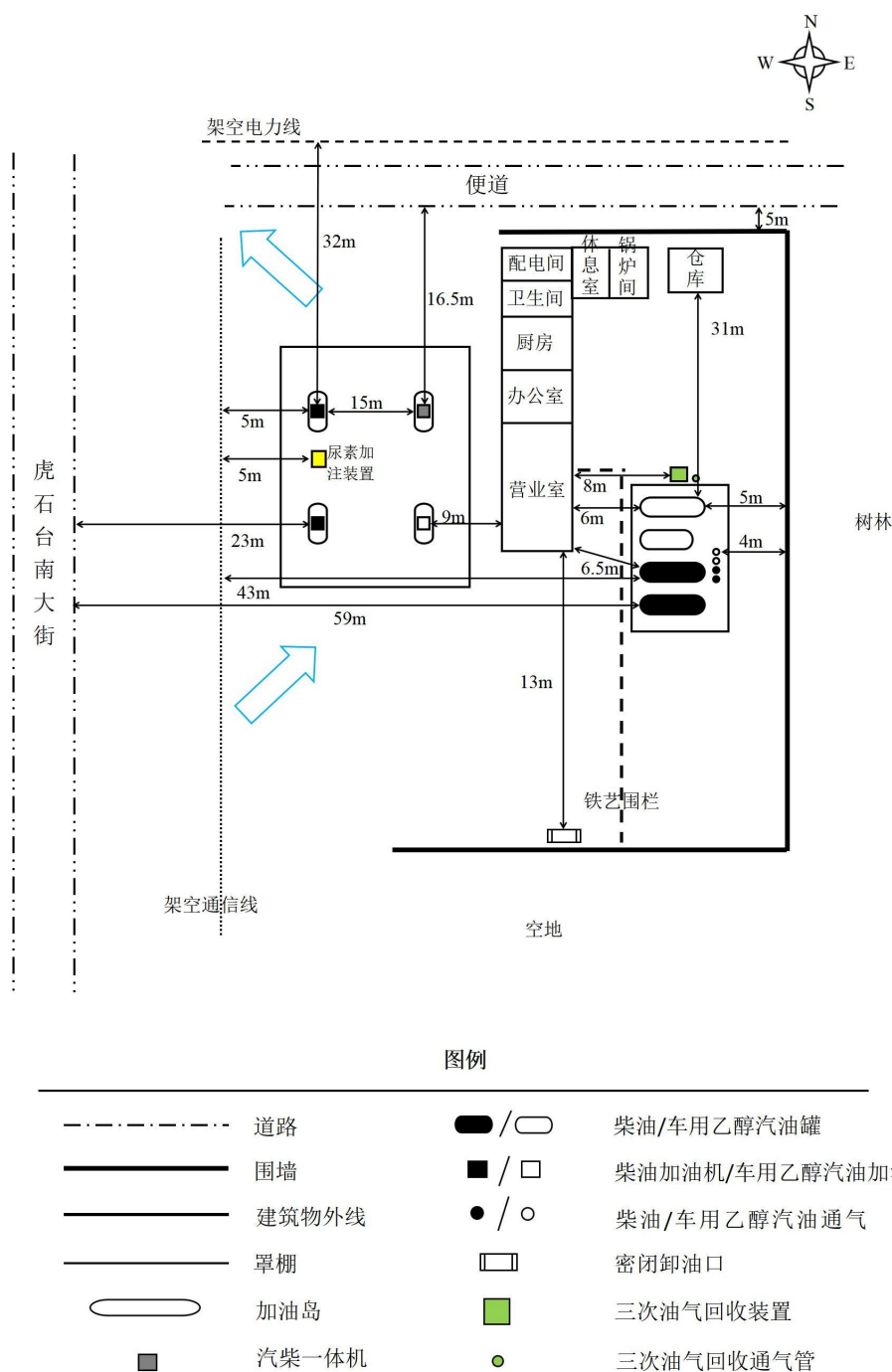
图 2.3-1 周边环境及总平面布置图
