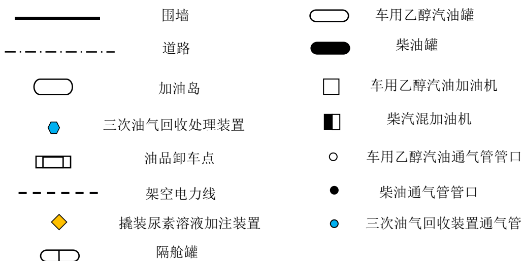
图 2.3-1 周边环境及总平面布置
