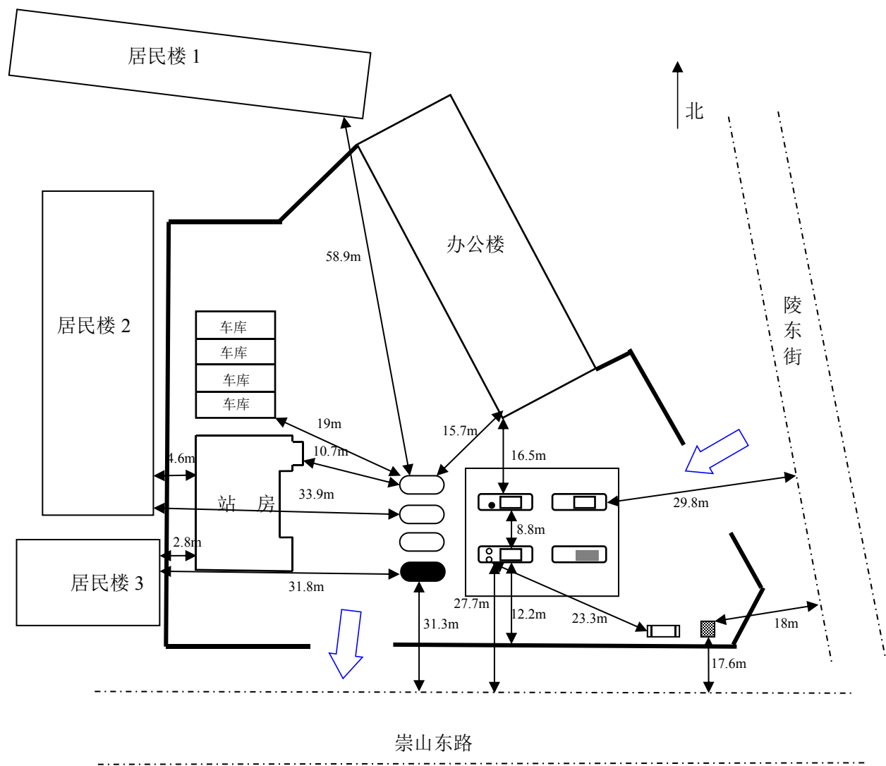
图 2.3-2 周边环境及总平面布置图
