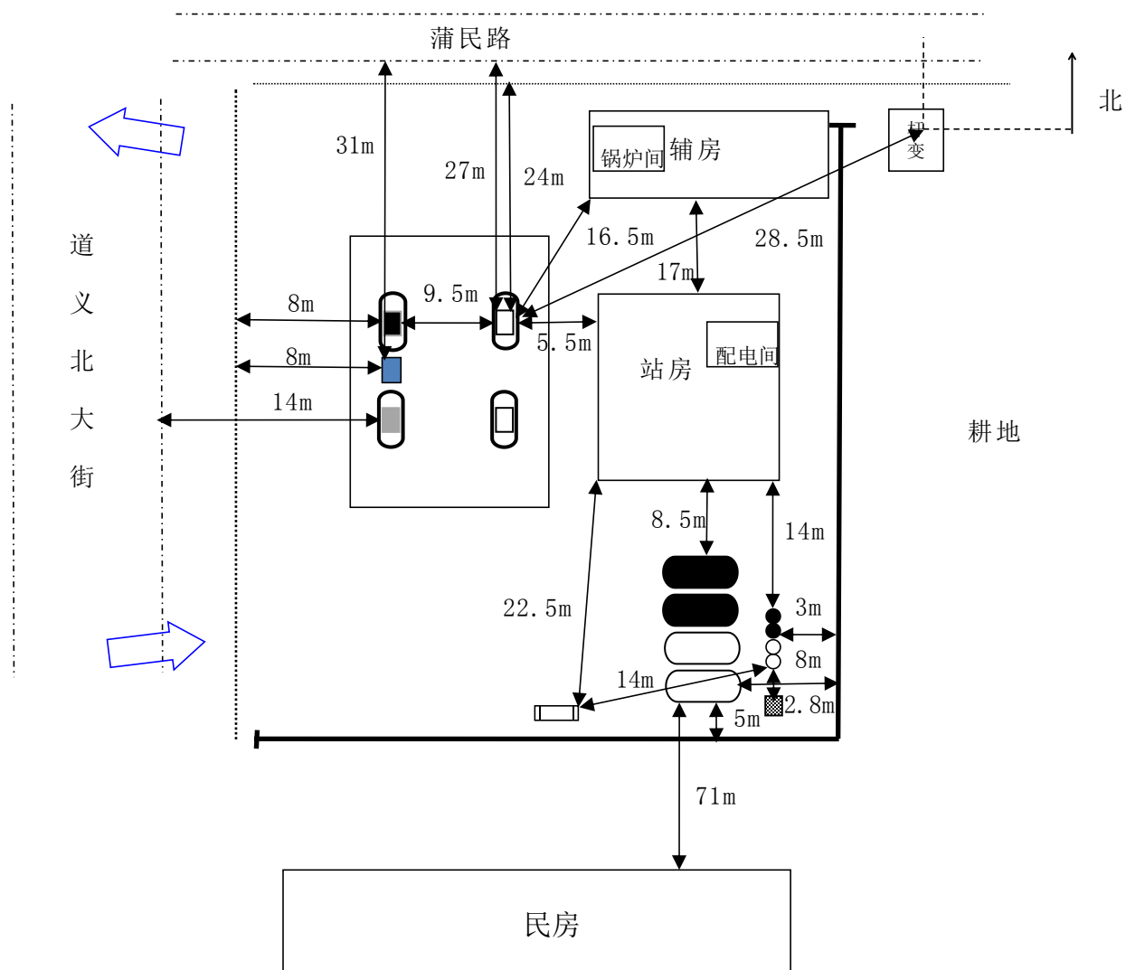
图 2-1 周边环境及总平面布置图
