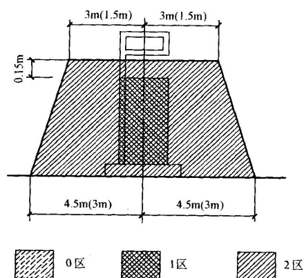
附图 1 汽油加油机爆炸危险区域划分
