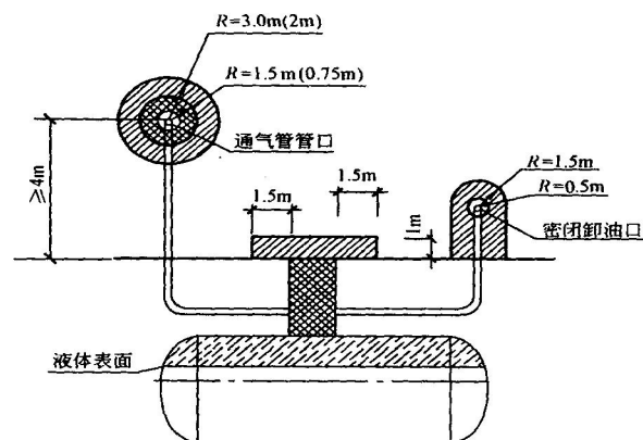
附图 3 埋地卧式汽油储罐爆炸危险区域划分
