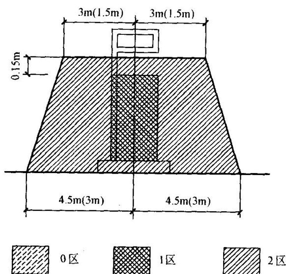
图 3.3-1 汽油加油机爆炸危险区域划分
