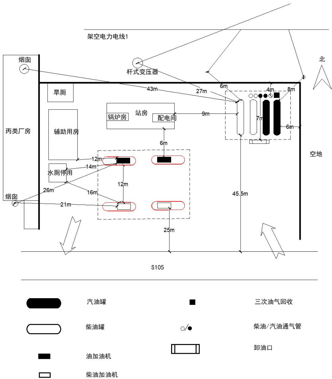
图 2.3-1 周边环境及总平面布置图
