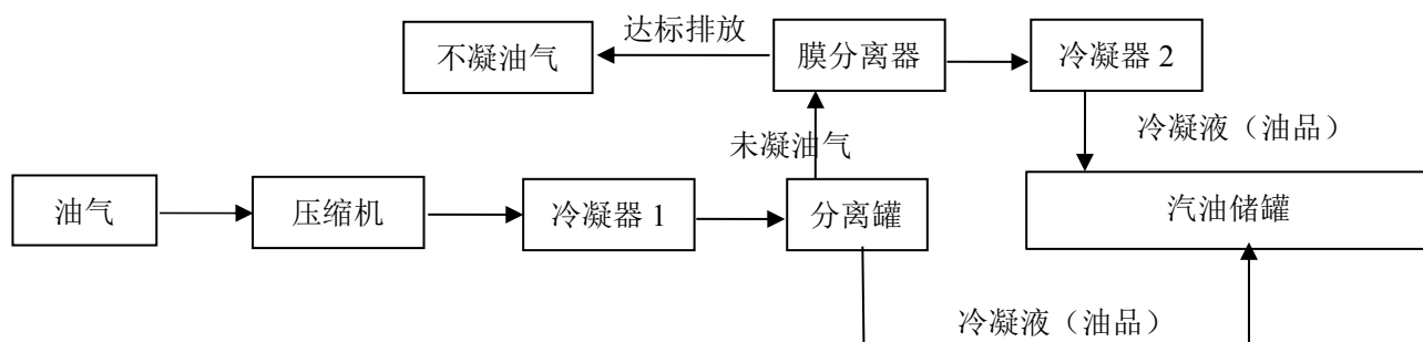
图 2-4 油气回收处理装置工艺流程框图（三次油气回收）
