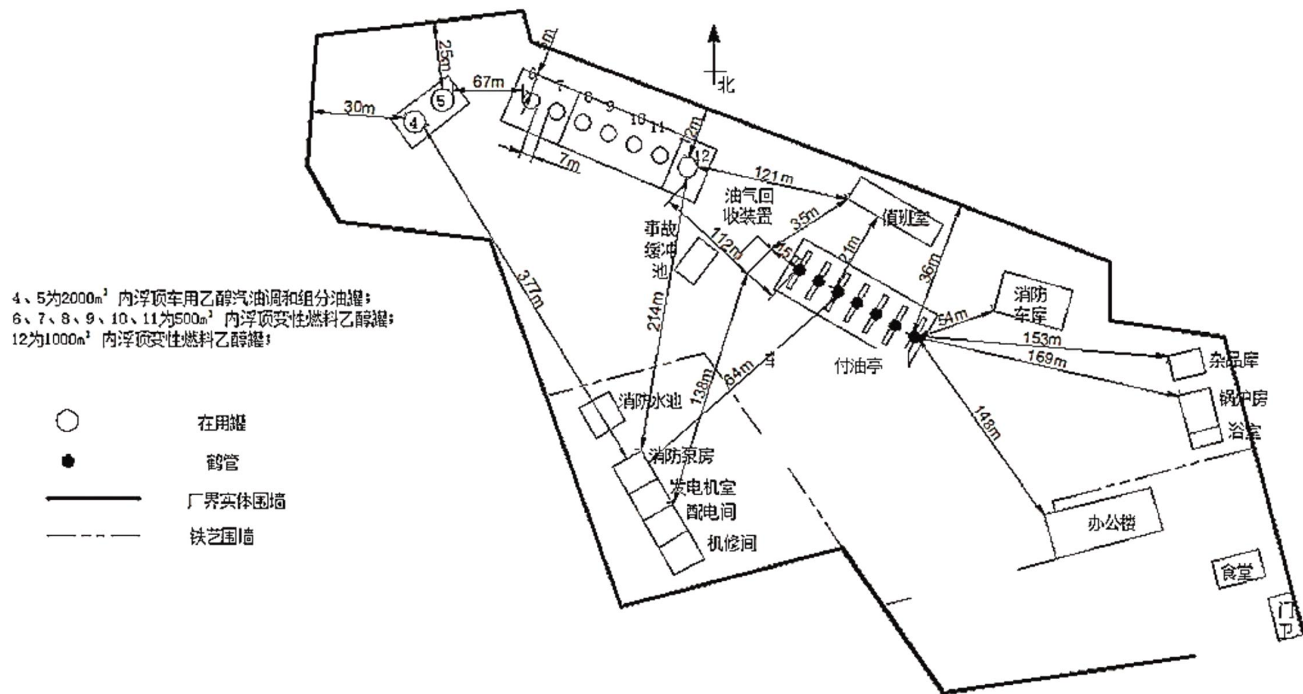
图 2-4 东陵油库北山储油区平面布置图
