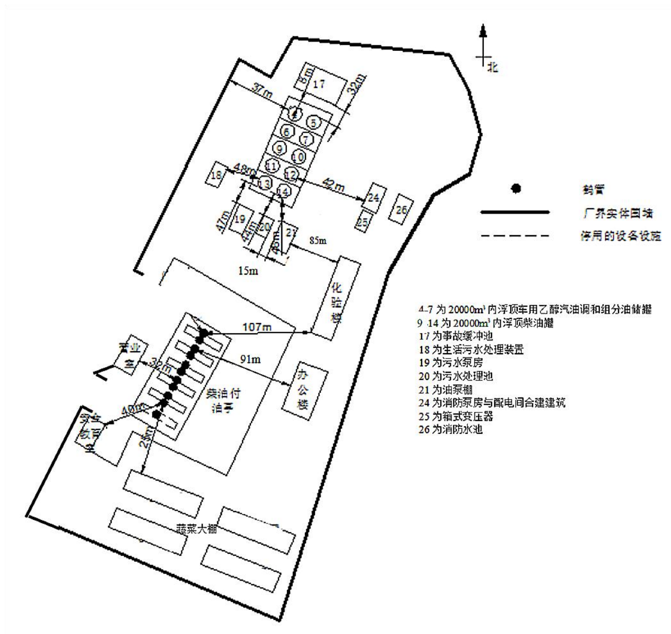
图 2-5 东陵油库东山储油区平面布置图
