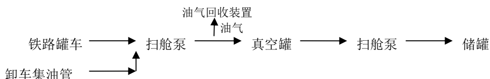
图 2-12 扫仓工艺流程示意图
