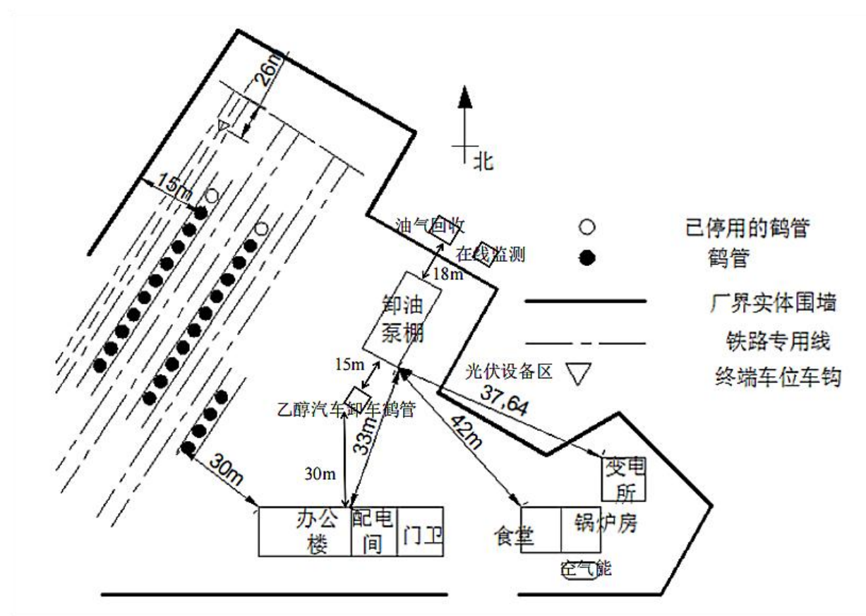
图 2-6 东陵油库铁路油品装卸区平面布置图
