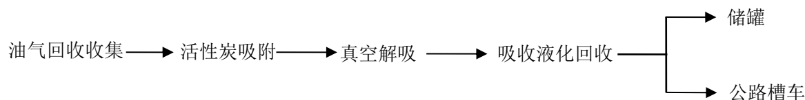
图 2-14 油气回收外网工艺流程示意图
