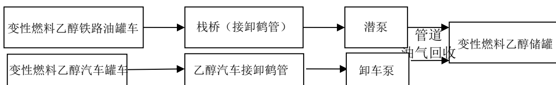
图 2-8 变性燃料乙醇接卸工艺流程示意框图
