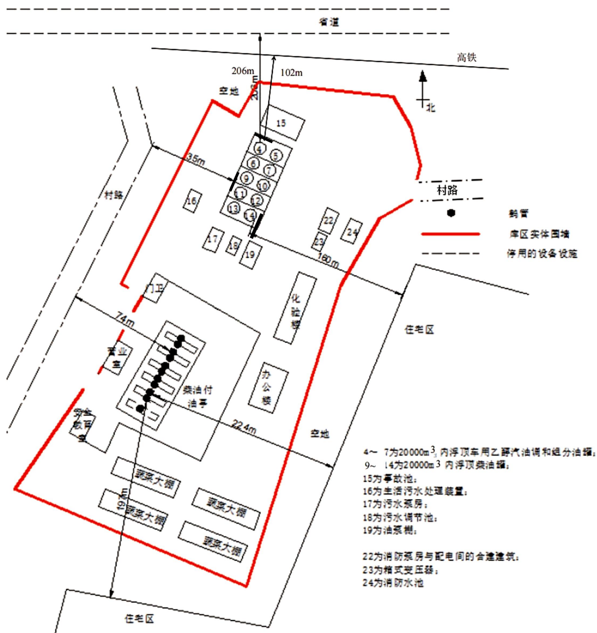
图 2-2 东陵油库东山储油区周边环境示意图
