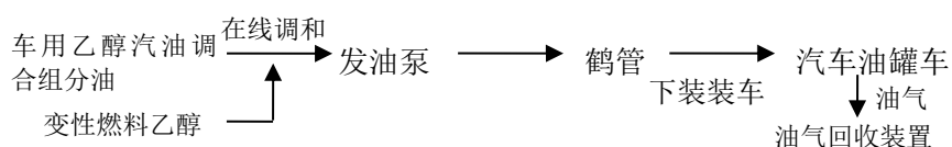
图 2-11 车用乙醇汽油公路装车工艺流程示意图
