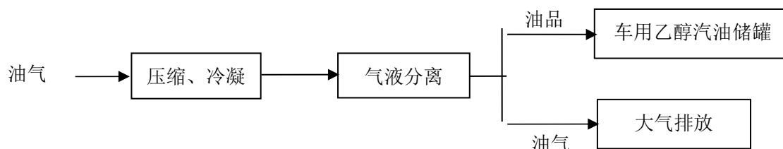
图 2-5 三次油气回收工艺流程框图
