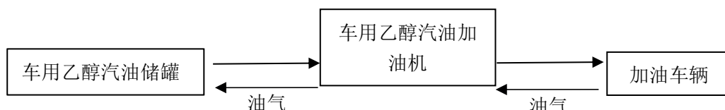
图 2.6-1 车用乙醇汽油加油工艺流程框图（二次油气回收）
