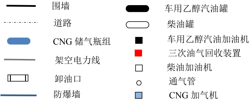
图 2-1 周边及总平面布置图
